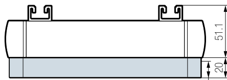
piastra spugna tipo "maxi"
