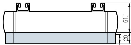
piastra spugna tipo "mini"
