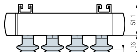
piastra ventose tipo "maxi"
